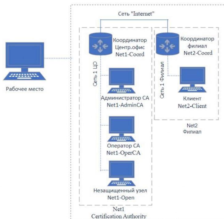
Рисунок 1 Схема защищенной сети
